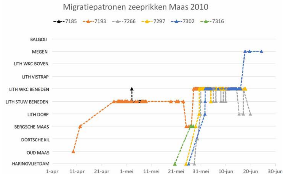
Het onderzoek laat zien dat de vispassages in de Maas in ieder geval tot aan de monding van de Roer optrekbaar zijn.
